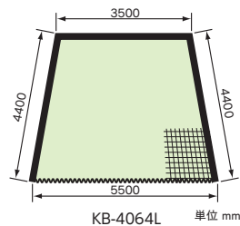
KB-4064のサイドフレーム 4.4m長タイプ
